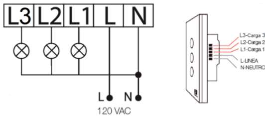
Conexión 110 Voltios
