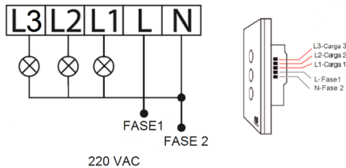
Conexión 220 Voltios
